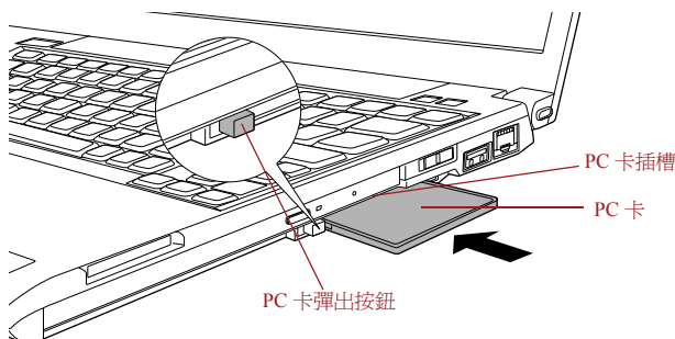
圖 3-1 插入 PC 卡
