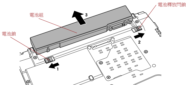
圖 6-1 釋放電池組
