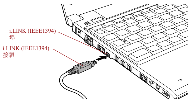
圖 3-12 將 i.LINK (IEEE1394) 纜線連線至電腦
