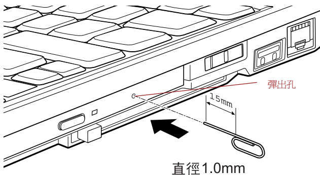
圖 4-7 使用彈出孔手動釋放托架
