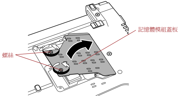
圖 3-5 移除記憶體模組蓋板
