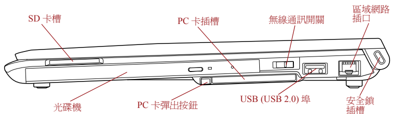
圖 2-3 電腦的右側
