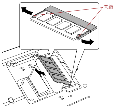
圖 3-8 移除記憶體模組
