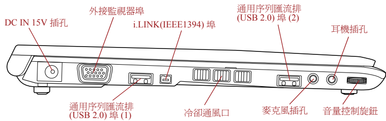
圖 2-2 電腦的左側
