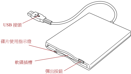
圖 3-10 USB 軟碟機
