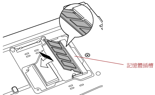
圖 3-6 記憶體模組就位
