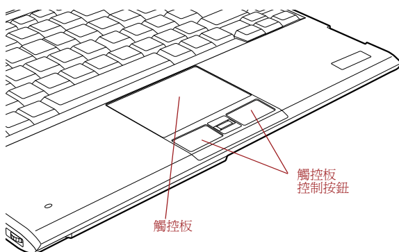
圖 4-1 觸控板與觸控板控制按鈕
