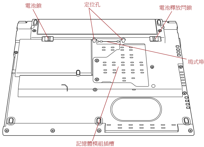
圖 2-5 電腦的底部
