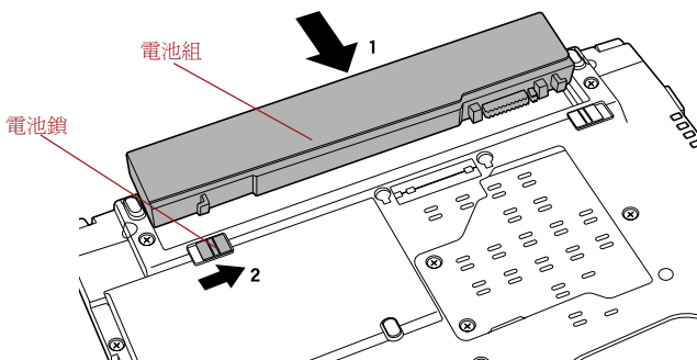
圖 6-2 固定電池組
