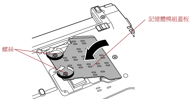
圖 3-7 記憶體模組蓋板就位
